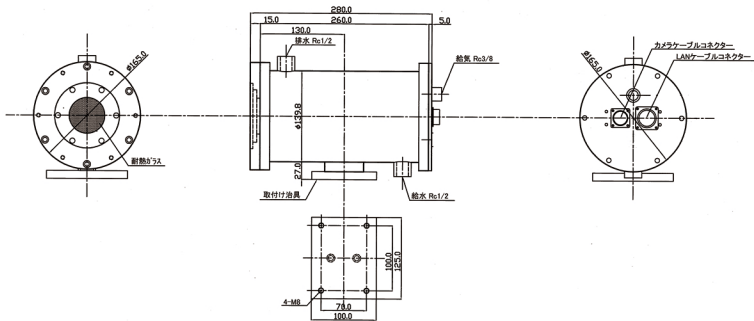
HRS-400RX/X外形寸法図
