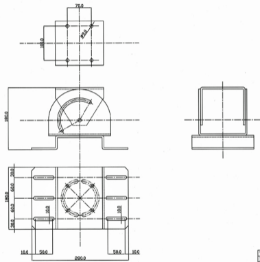
MU-01 舞台外形図
